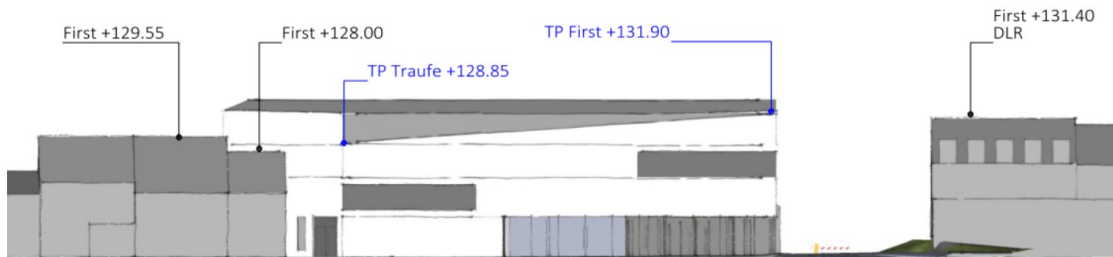
Skizze als Ansicht von der Gartenstraße mit Höhenvergleich zur Nachbarbebauung
